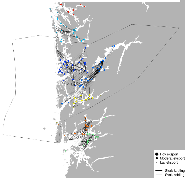
PO3 - Modellert konektivitet i perioden 2025-05-13 - 2025-05-23
