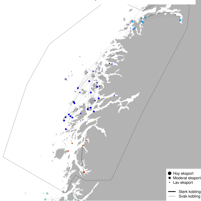
PO8 - Modellert konnektivitet i perioden 2025-05-13 - 2025-05-23
