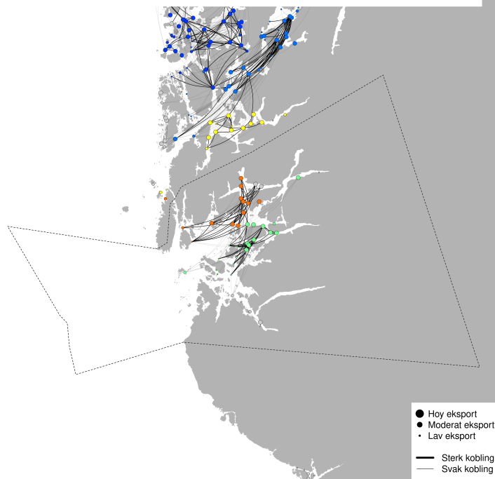
PO2 - Modellert konektivitet i perioden 2025-05-13 - 2025-05-23
