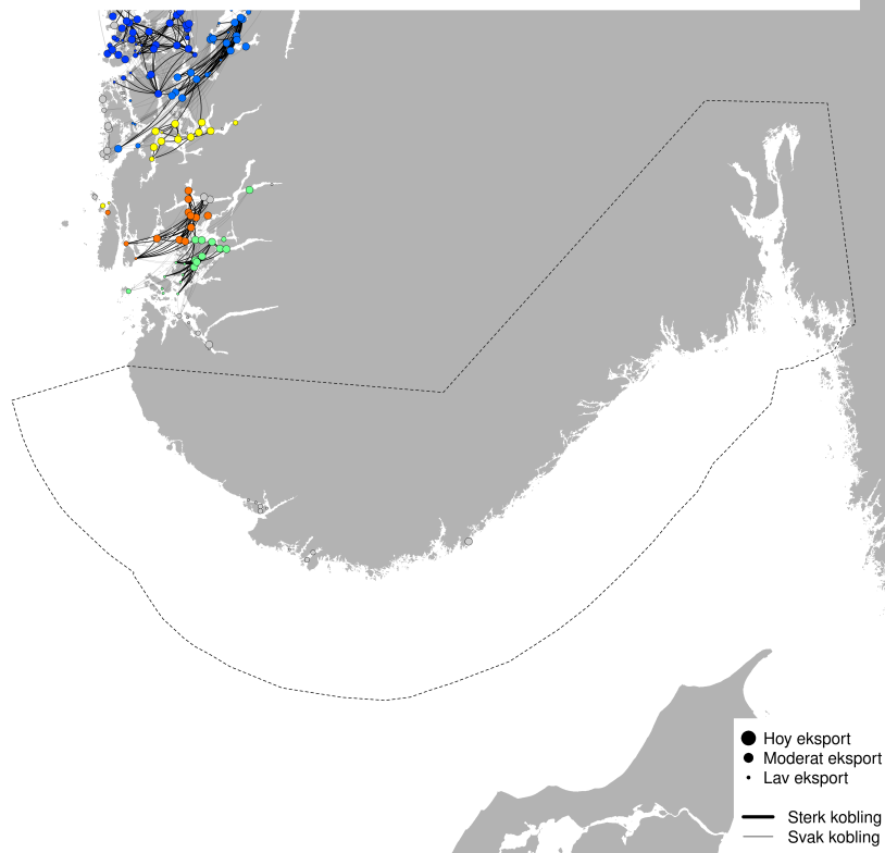
PO1 - Modellert konnektivitet i perioden 2025-05-13 - 2025-05-23
