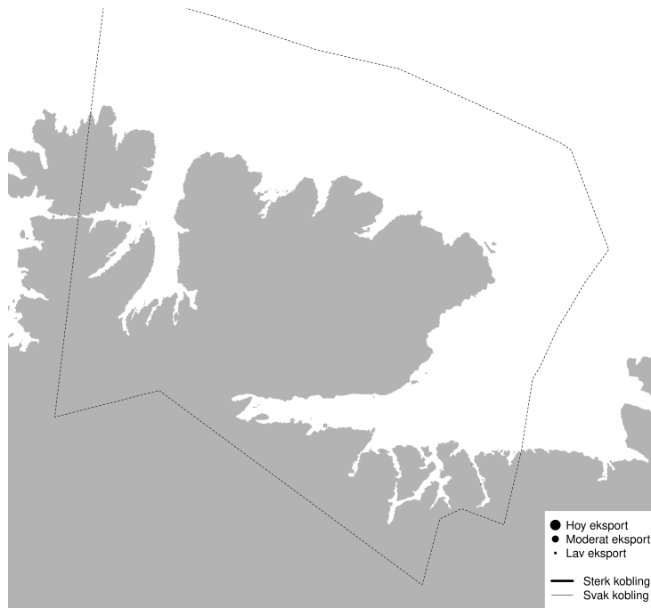
PO13 - Modellert konnektivitet i perioden 2025-05-13 - 2025-05-23
