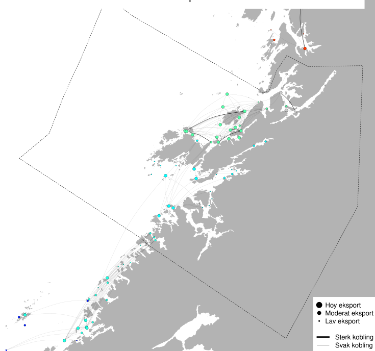
PO7 - Modellert konnektivitet i perioden 2025-05-13 - 2025-05-23
