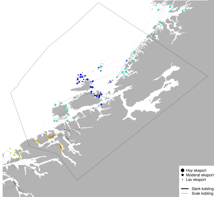
PO6 - Modellert konnektivitet i perioden 2025-05-13 - 2025-05-23
