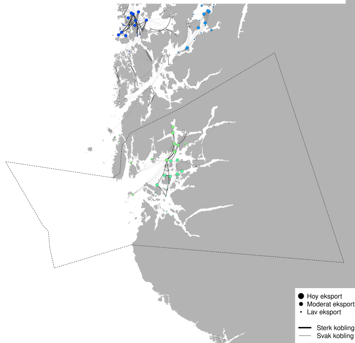
PO2 - Modellert konektivitet i perioden 2025-07-22 - 2025-08-01
