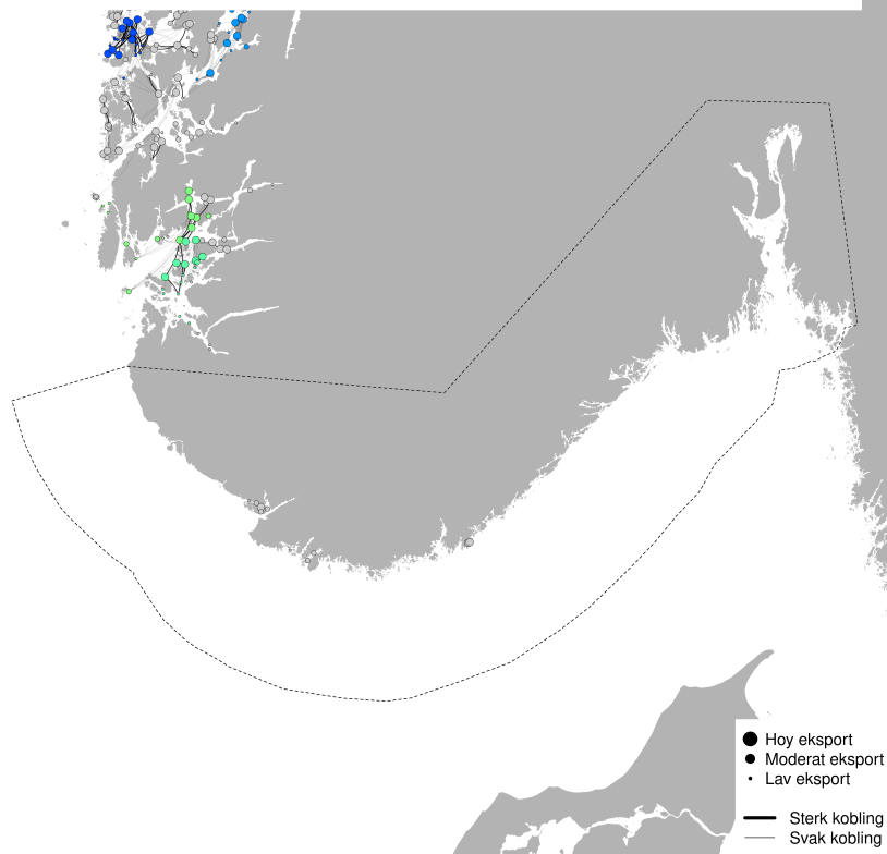
PO1 - Modellert konnektivitet i perioden 2025-07-22 - 2025-08-01
