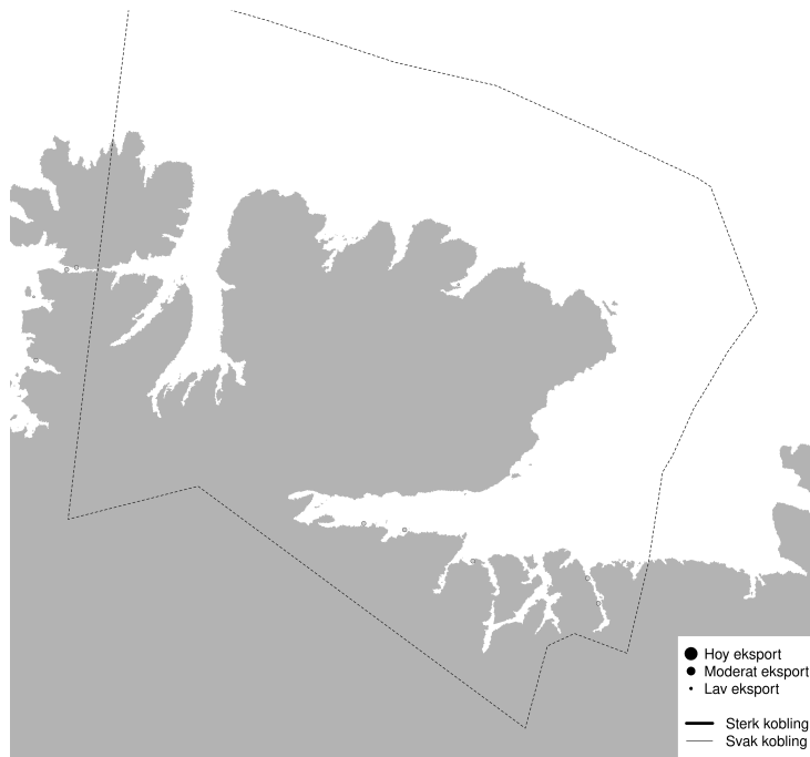
PO13 - Modellert konnektivitet i perioden 2025-07-22 - 2025-08-01
