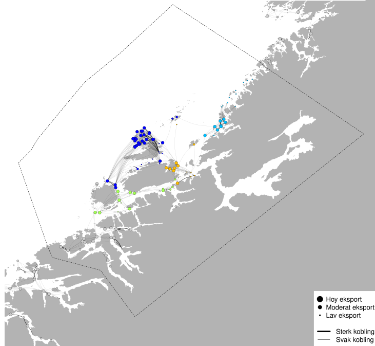
PO6 - Modellert konnektivitet i perioden 2025-07-22 - 2025-08-01
