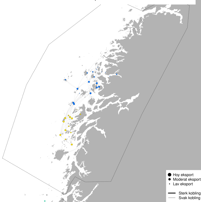
PO8 - Modellert konnektivitet i perioden 2025-07-22 - 2025-08-01
