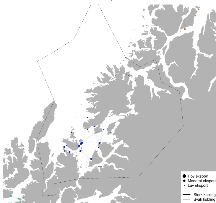
PO10 - Modellert konnektivitet i perioden 2025-07-22 - 2025-08-01
