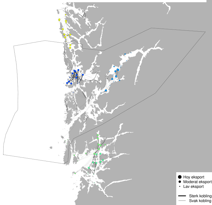
PO3 - Modellert konektivitet i perioden 2025-07-22 - 2025-08-01
