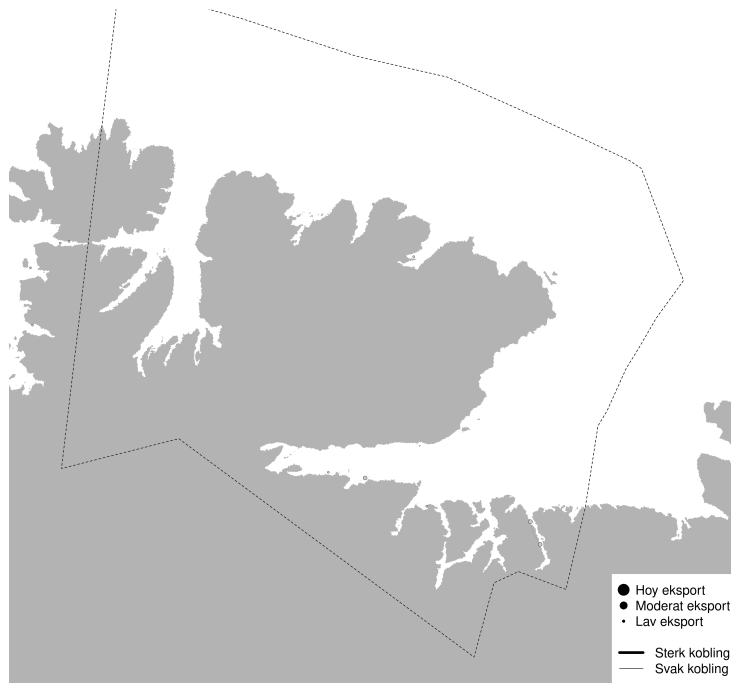
PO13 - Modellert konnektivitet i perioden 2025-09-09 - 2025-09-19
