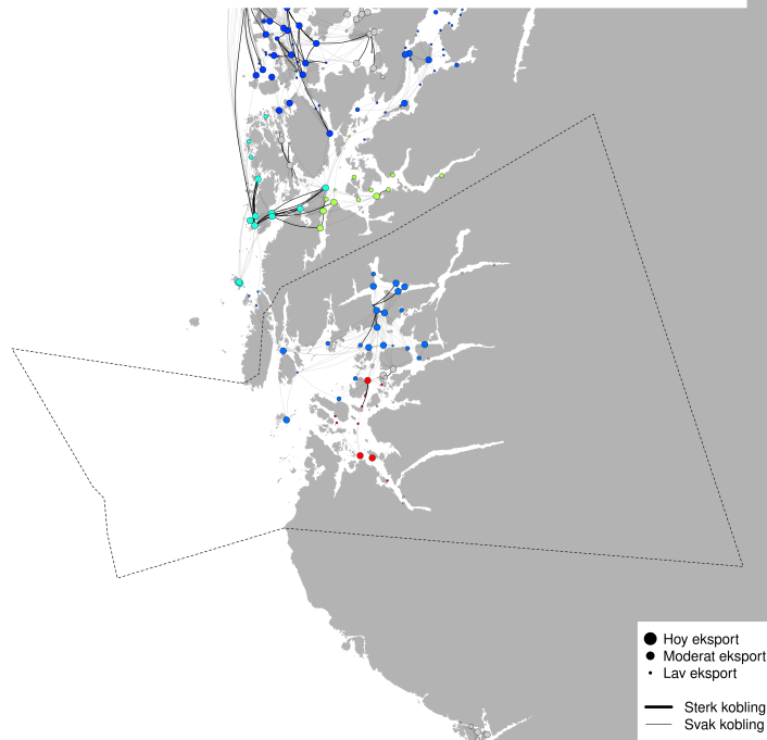
PO2 - Modellert konektivitet i perioden 2025-09-09 - 2025-09-19
