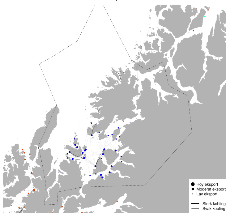
PO10 - Modellert konektivitet i perioden 2025-09-09 - 2025-09-19
