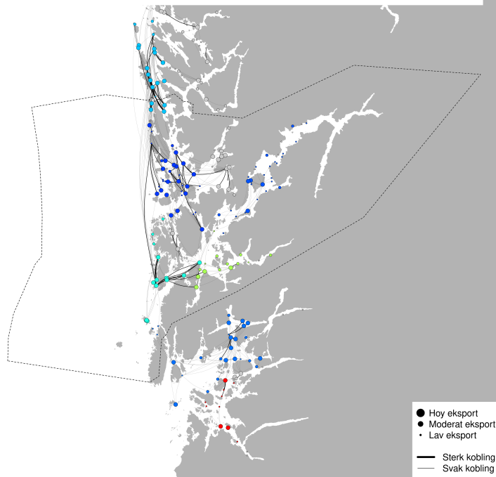
PO3 - Modellert konektivitet i perioden 2025-09-09 - 2025-09-19
