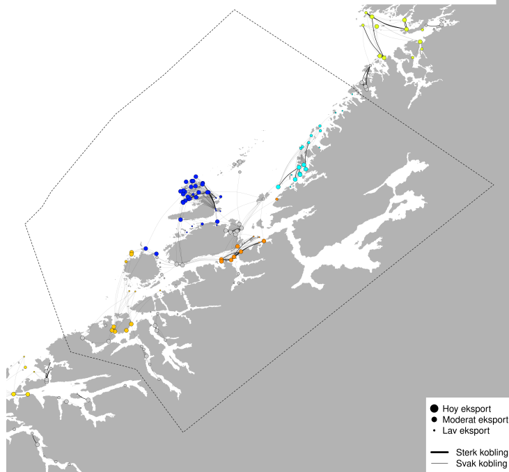
PO6 - Modellert konnektivitet i perioden 2025-09-09 - 2025-09-19
