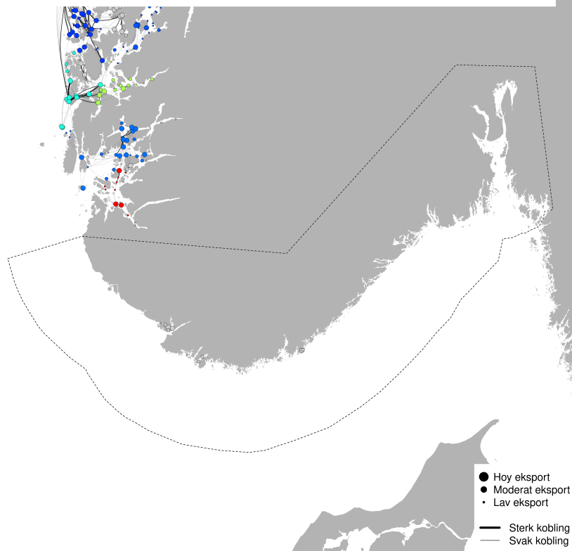
PO1 - Modellert konnektivitet i perioden 2025-09-09 - 2025-09-19
