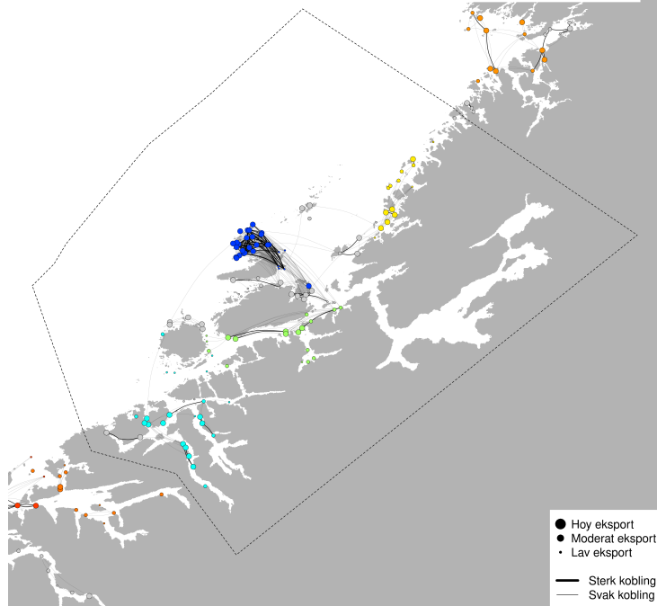
PO6 - Modellert konnektivitet i perioden 2025-09-23 - 2025-10-03
