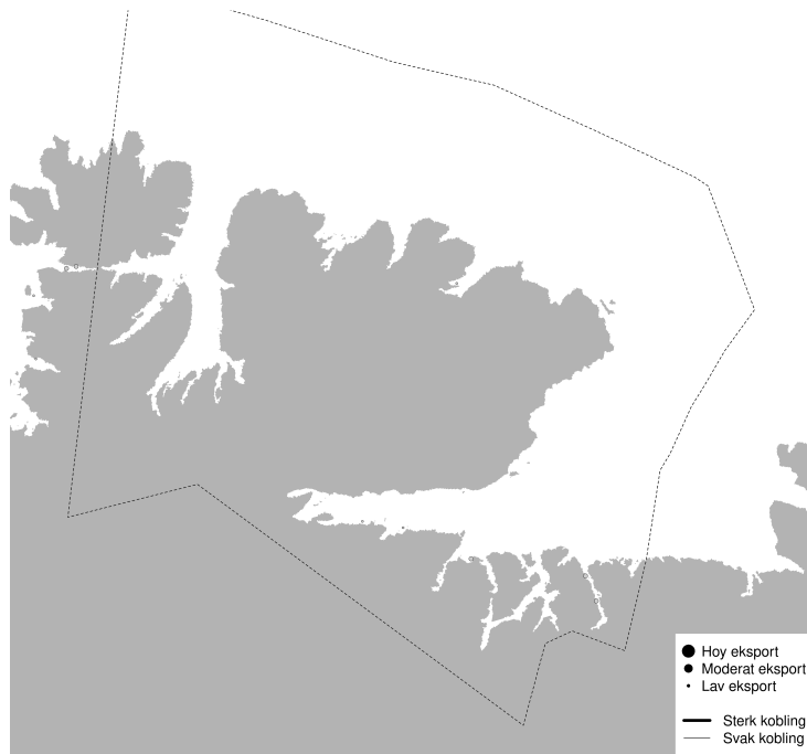
PO13 - Modellert konnektivitet i perioden 2025-09-23 - 2025-10-03
