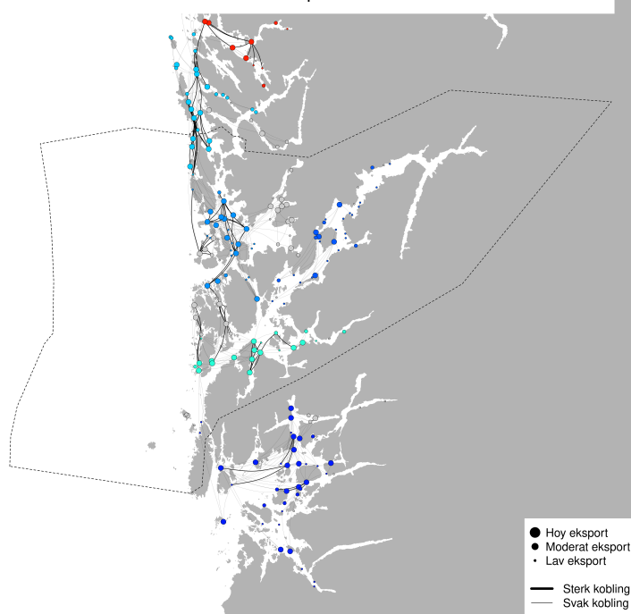
PO3 - Modellert konektivitet i perioden 2025-09-23 - 2025-10-03
