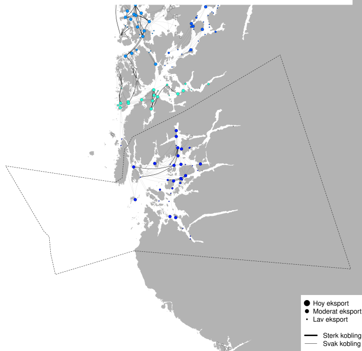
PO2 - Modellert konektivitet i perioden 2025-09-23 - 2025-10-03
