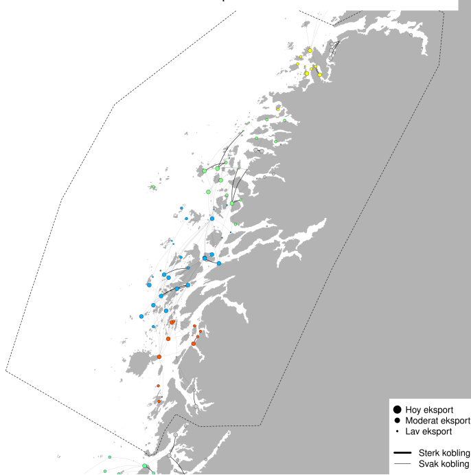
PO8 - Modellert konnektivitet i perioden 2025-09-23 - 2025-10-03
