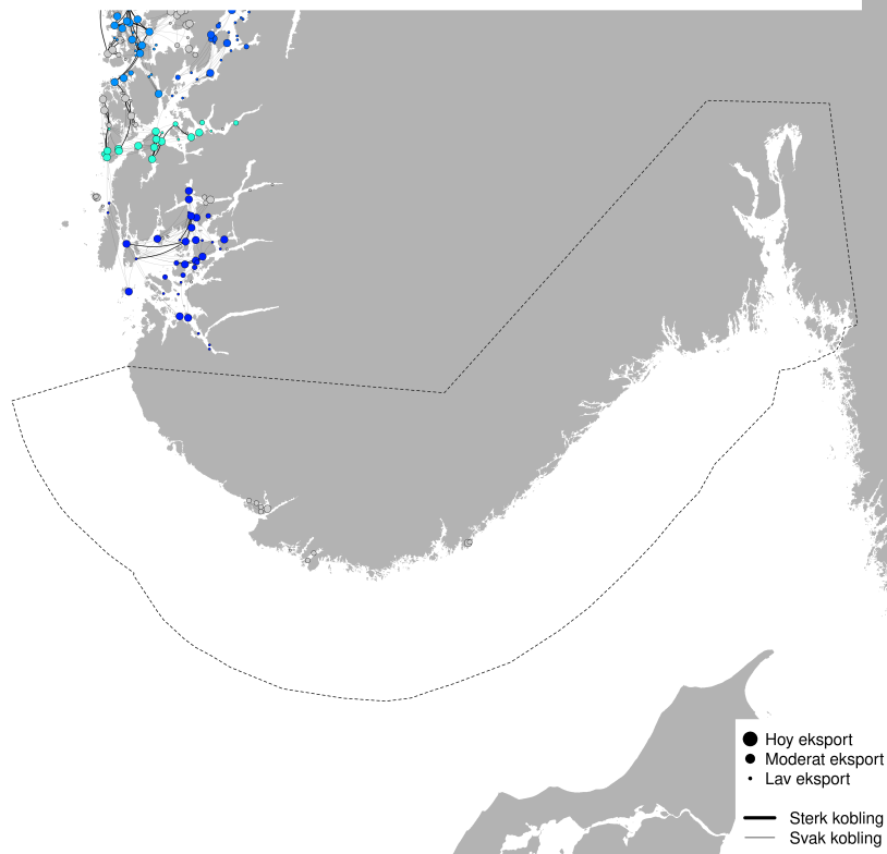
PO1 - Modellert konnektivitet i perioden 2025-09-23 - 2025-10-03
