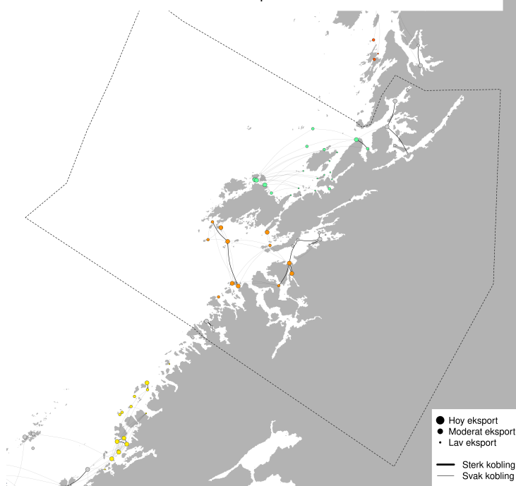
PO7 - Modellert konektivitet i perioden 2025-09-23 - 2025-10-03
