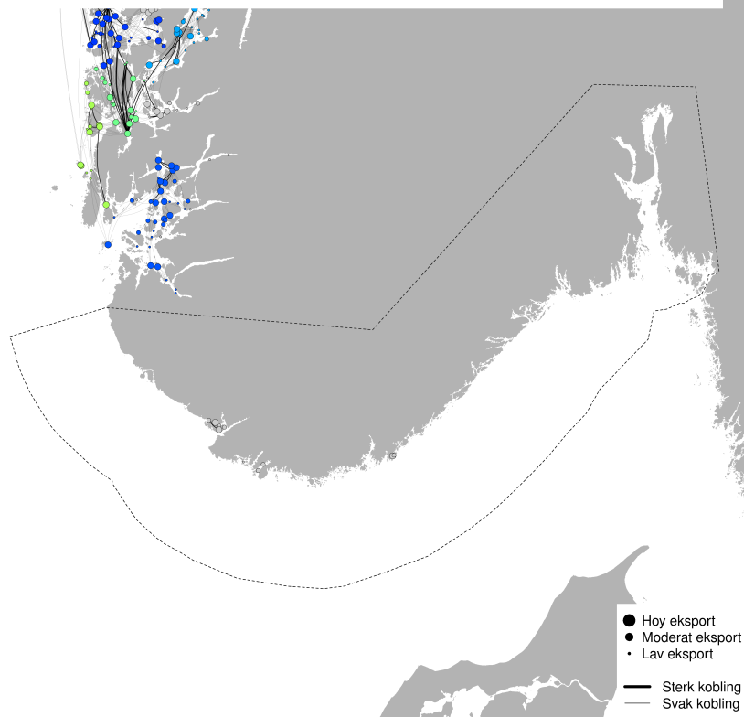
PO1 - Modellert konnektivitet i perioden 2025-10-02 - 2025-10-12
