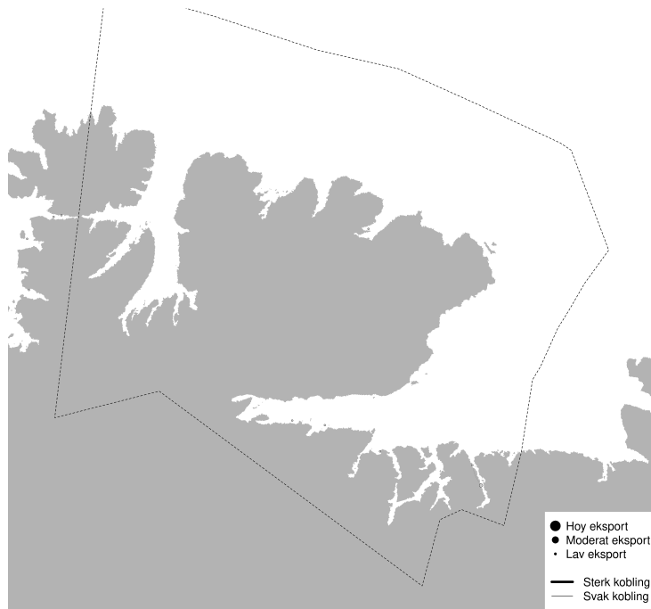
PO13 - Modellert konnektivitet i perioden 2025-10-02 - 2025-10-12
