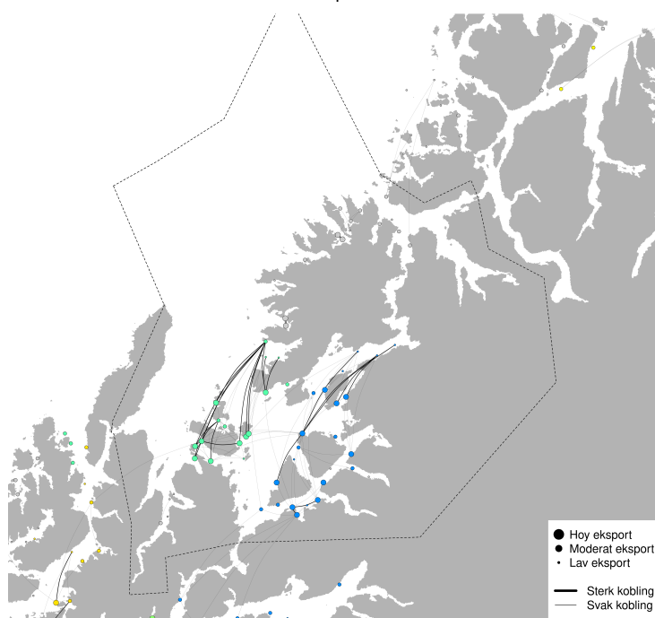
PO10 - Modellert konnektivitet i perioden 2025-10-02 - 2025-10-12
