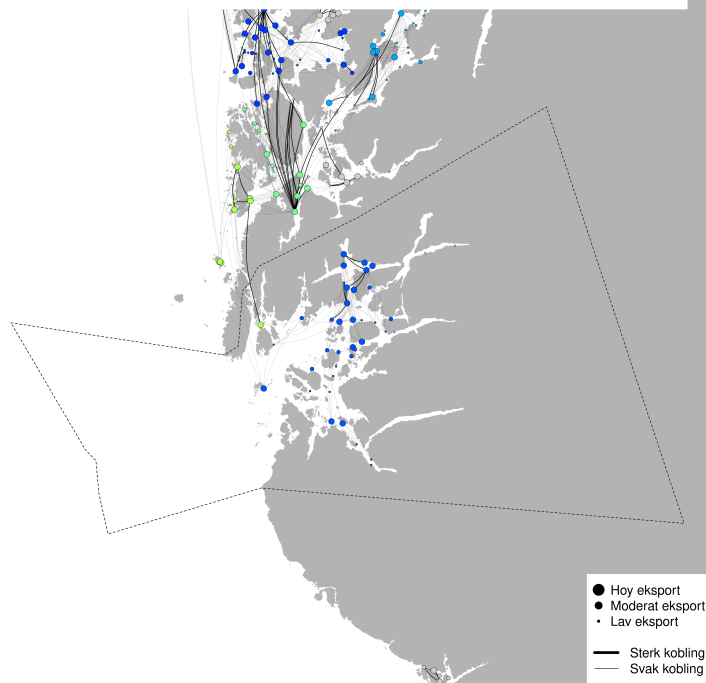
PO2 - Modellert konektivitet i perioden 2025-10-02 - 2025-10-12
