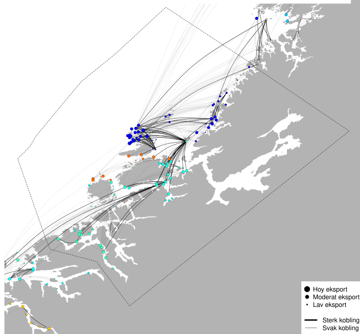
PO6 - Modellert konnektivitet i perioden 2025-10-02 - 2025-10-12
