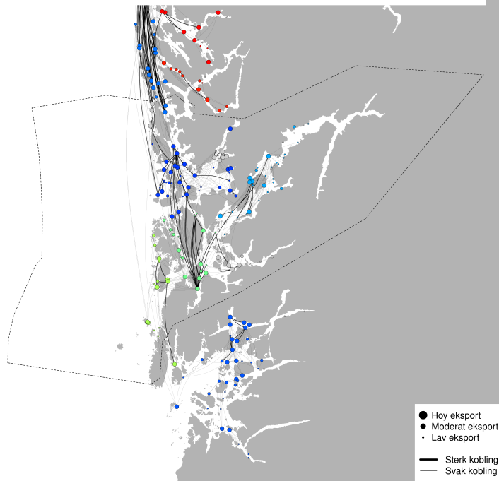
PO3 - Modellert konektivitet i perioden 2025-10-02 - 2025-10-12
