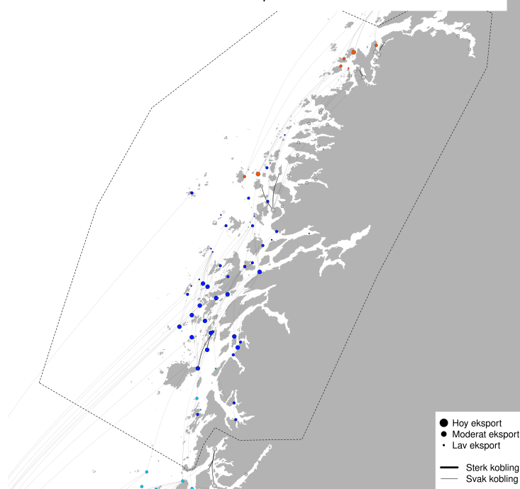
PO8 - Modellert konnektivitet i perioden 2025-10-02 - 2025-10-12
