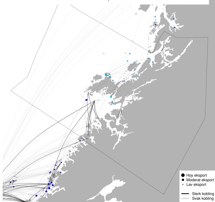
PO7 - Modellert konektivitet i perioden 2025-10-02 - 2025-10-12
