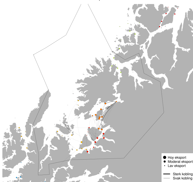
PO10 - Modellert konnektivitet i perioden 2026-01-15 - 2026-01-25
