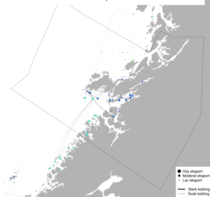
PO7 - Modellert konnektivitet i perioden 2026-01-15 - 2026-01-25
