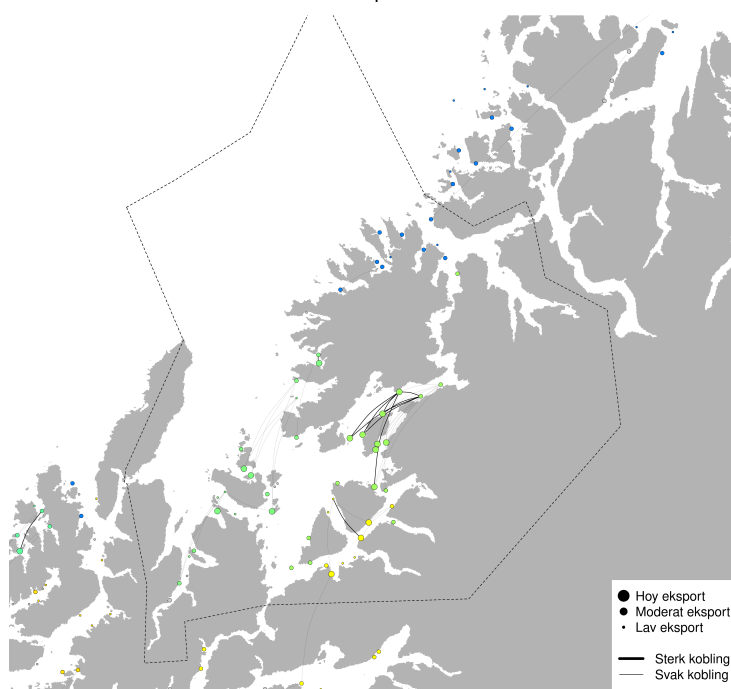
PO10 - Modellert konektivitet i perioden 2026-03-05 - 2026-03-15
