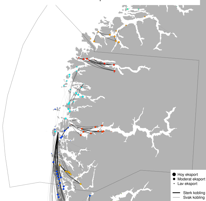
PO4 - Modellert konnektivitet i perioden 2026-03-05 - 2026-03-15
