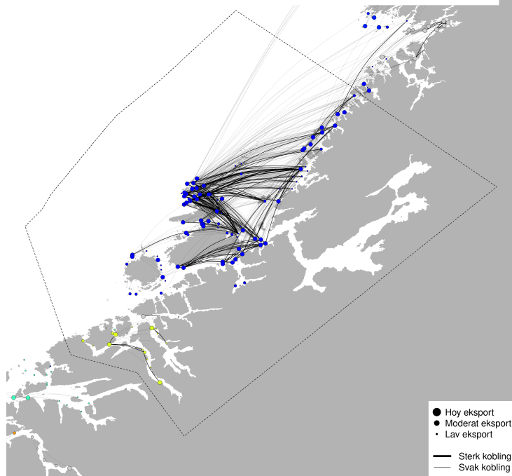
PO6 - Modellert konnektivitet i perioden 2026-03-05 - 2026-03-15
