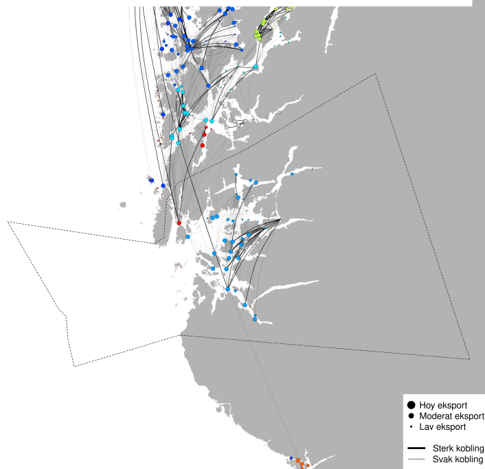
PO2 - Modellert konektivitet i perioden 2026-03-05 - 2026-03-15
