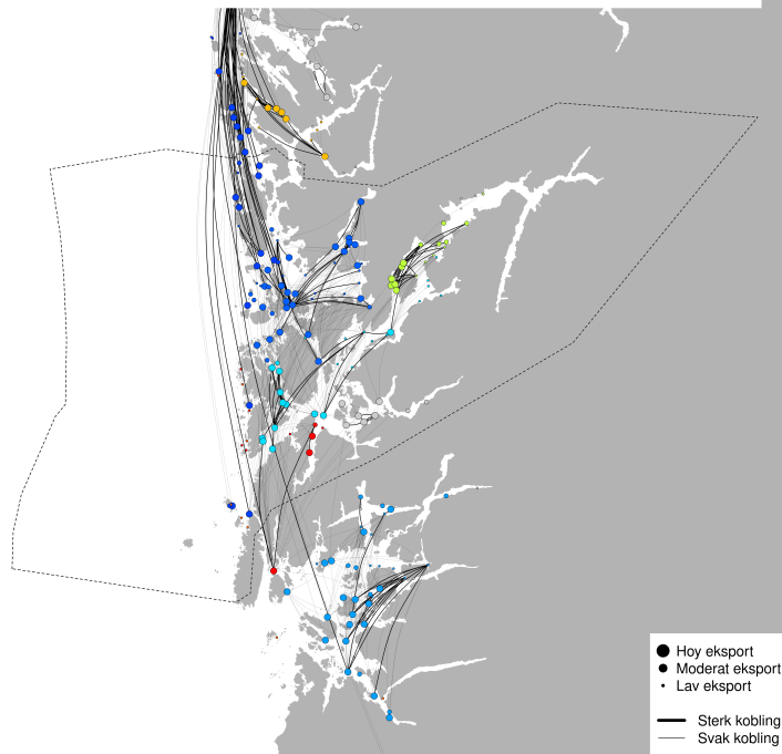
PO3 - Modellert konektivitet i perioden 2026-03-05 - 2026-03-15
