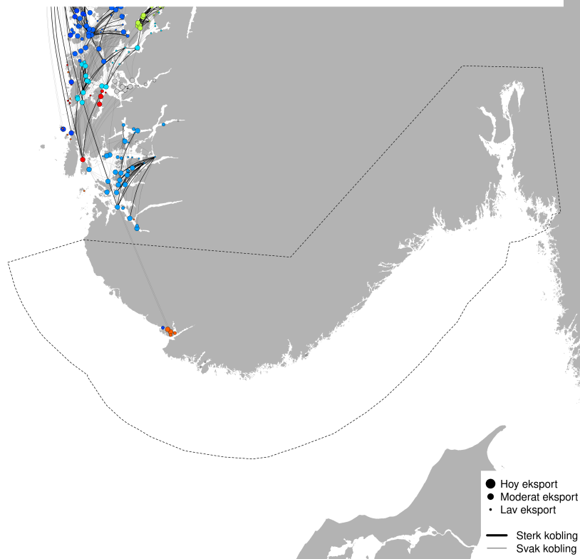
PO1 - Modellert konnektivitet i perioden 2026-03-05 - 2026-03-15
