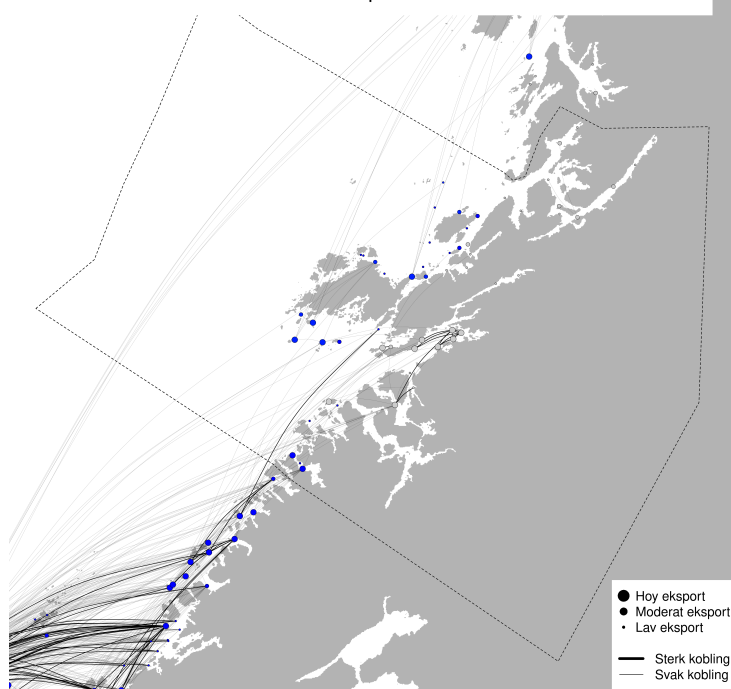
PO7 - Modellert konektivitet i perioden 2026-03-05 - 2026-03-15
