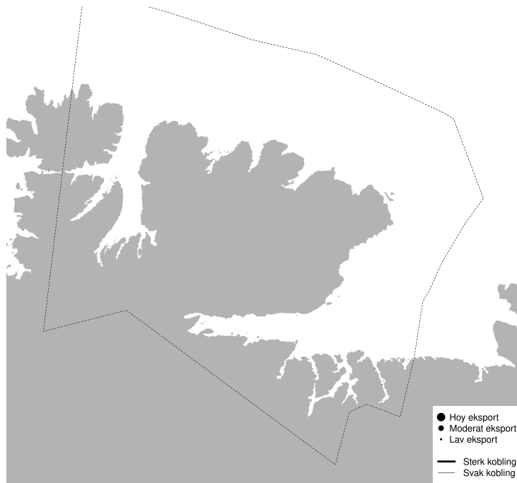
PO13 - Modellert konnektivitet i perioden 2026-03-05 - 2026-03-15
