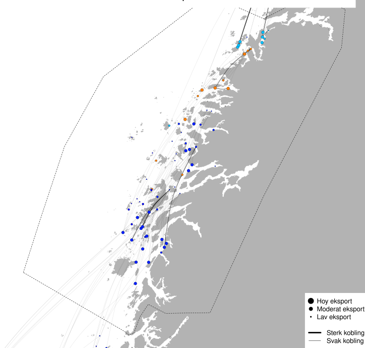
PO8 - Modellert konnektivitet i perioden 2026-03-05 - 2026-03-15
