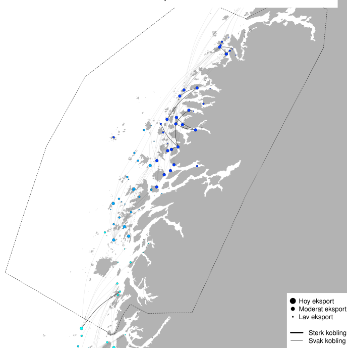
PO8 - Modellert konnektivitet i perioden 2026-07-30 - 2026-08-09
