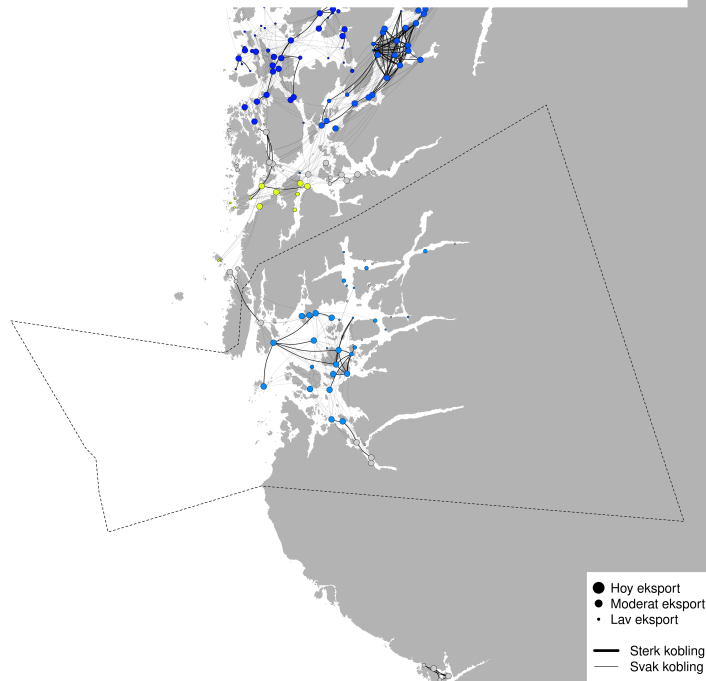
PO2 - Modellert konektivitet i perioden 2026-07-30 - 2026-08-09
