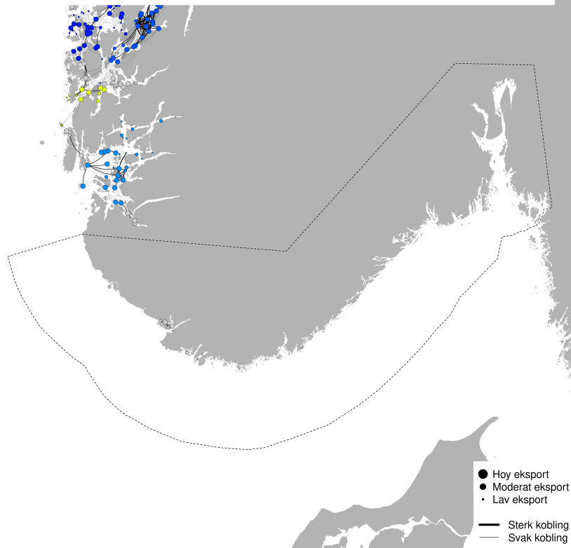
PO1 - Modellert konnektivitet i perioden 2026-07-30 - 2026-08-09
