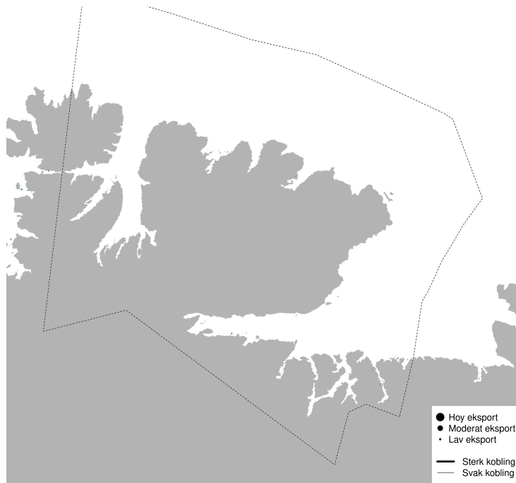
PO13 - Modellert konnektivitet i perioden 2026-07-30 - 2026-08-09
