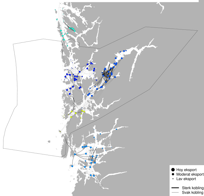
PO3 - Modellert konektivitet i perioden 2026-07-30 - 2026-08-09
